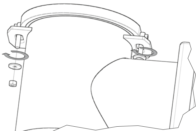
KROK 1. Odkręcić nakrętki mocujące płytę palnika retortowego.
