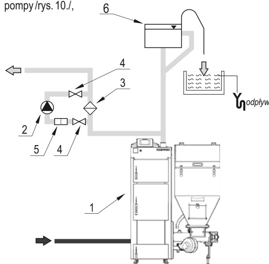
Rysunek 10. Wykonanie obejścia grawitacyjnego: 1-kocioł; 2-pompa obiegowa; 3-zawór różnicowy; 4-zawory odcinające; 5-filtr; 6-otwarte naczynia wzbiorcze.
