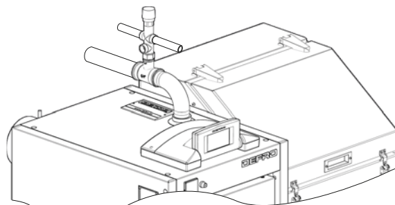
Rysunek 9. Przykładowy sposób podłączenia zaworu DBV-2.
