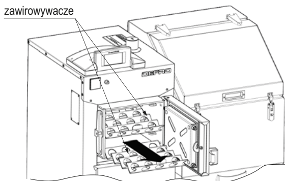
KROK 4. Ostrożnie wysunąć zawirowywacze. Oczyszczyć zawirowywacze oraz powierzchnię wymiany ciepła. Zamontować w odwrotnej kolejności
