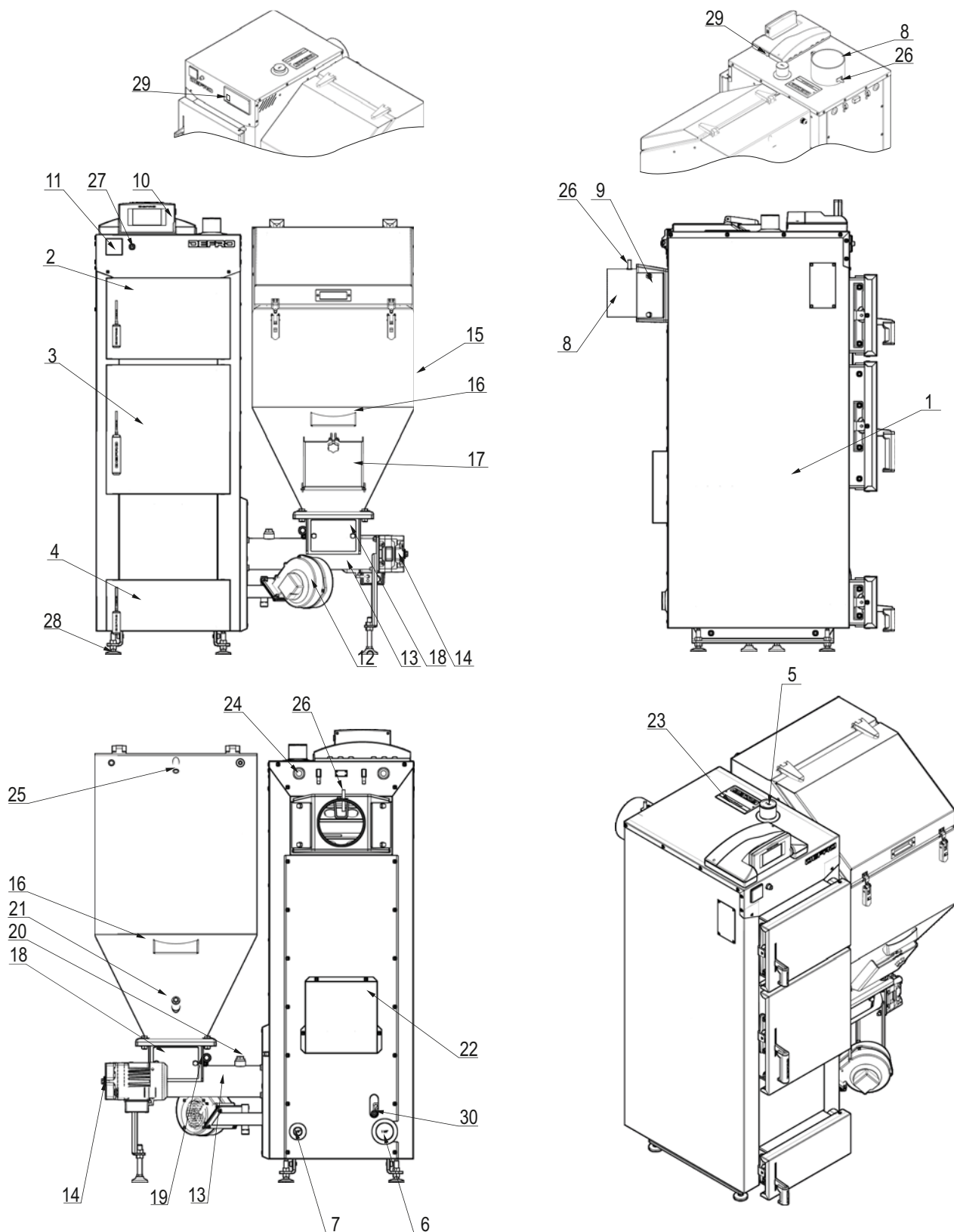
Rysunek 3. Podstawowe elementy kotłów.
