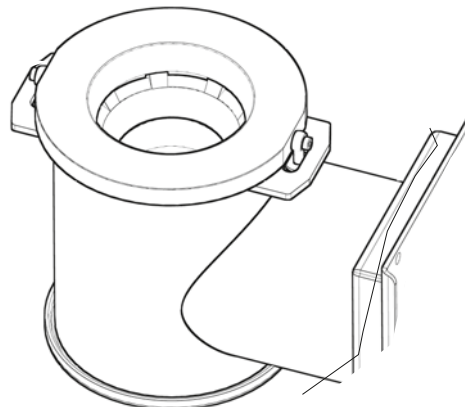
KROK 5. Poprawnie zmontowany palnik retortowy z wycelowaną płytą i koroną paleniska
