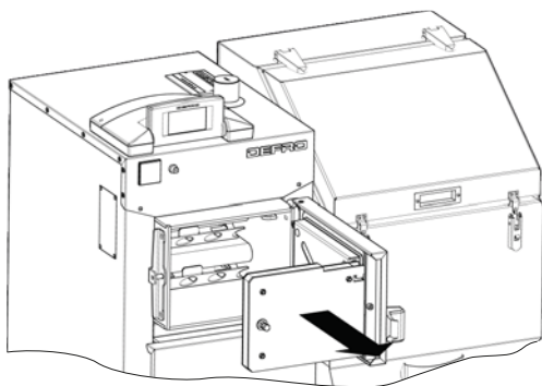
KROK 3. Wyjąć z kotła drzwi odbojnicowe.
