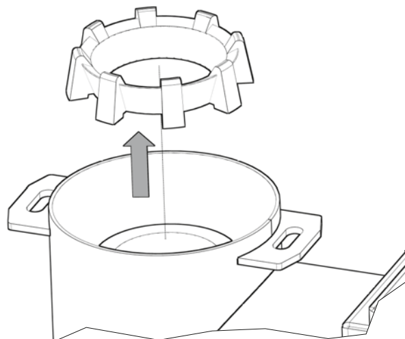
KROK 3. Zdjąć koronę palnika retortowego.
