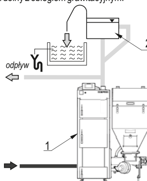
Rysunek 6. Przykładowy schemat zabezpieczeń kotła w układzie otwartym: 1-kocioł; 2-otwarte naczynie wzbiorcze.
