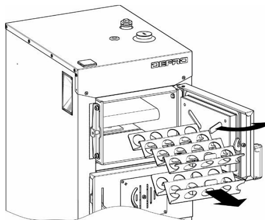
KROK 1. Otworzyć drzwi wyczystne. Wyjąć dolny i środkowy zaworowycze.
