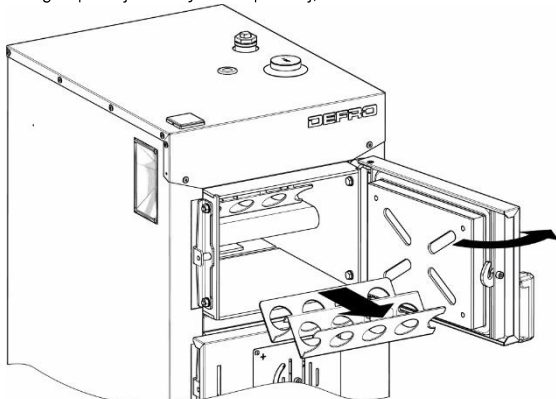
KROK 1. Otworzyć drzwi wyczystnie i wyjąć dolny zaworowywacz.
