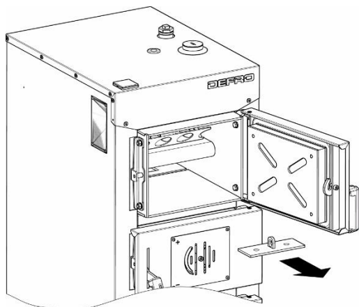
KROK 2. Wyjąć kłapkę krótkiego obiegu.
