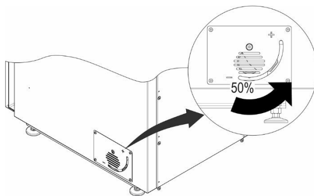
Rysunek 13. Prawidłowe położenie przepustnicy powietrza wtórnego dyszy w czasie.
