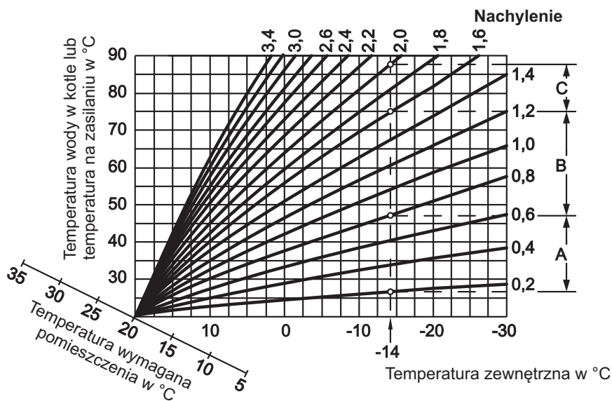
Rys. 9 Krzywe grzewcze
