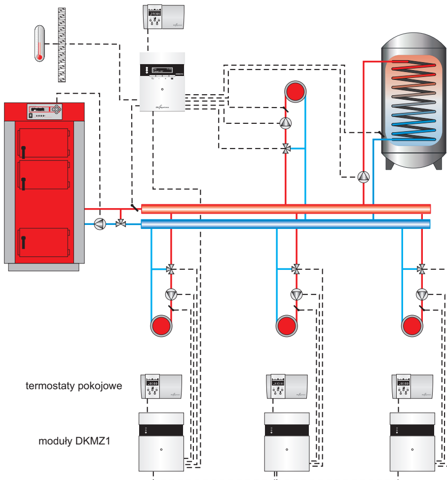
Rys. 17 Przykładowy schemat instalacji z podłączonymi trzema modułami rozszerzającymi DKMZ : Obiegu 3 , Obiegu 4 i Obiegu 5 .
