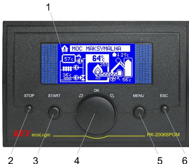
Rysunek 1. Płyta czołowa regulatora RK-2006SPGM.
