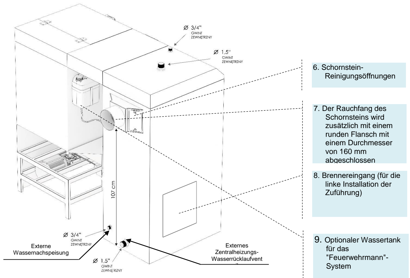
Abb. 4. Grundlegende Gesamtabmessungen des Kessels - seitliche Rückansicht.
