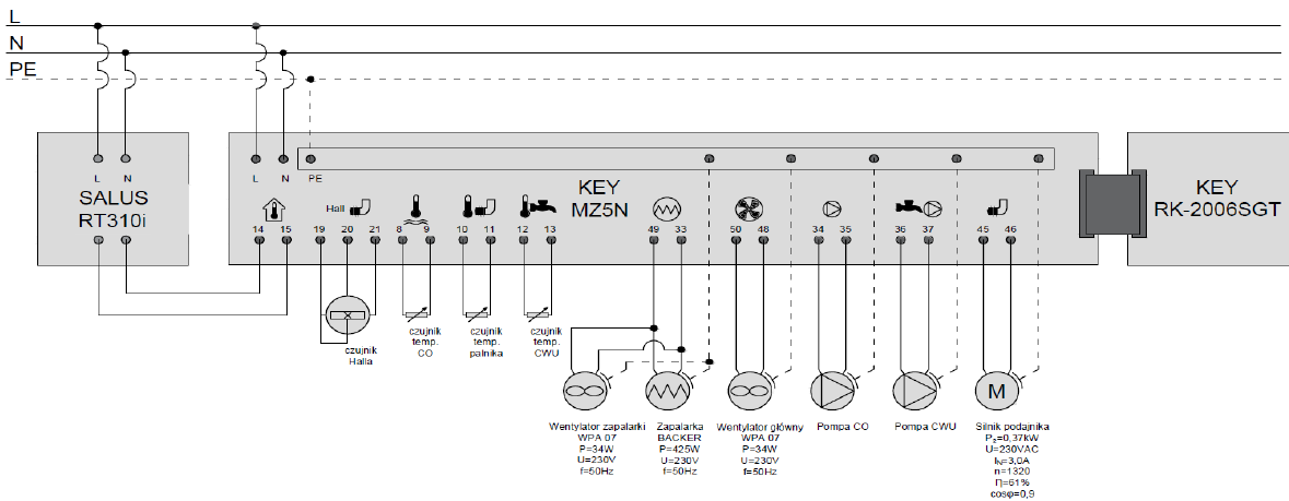
Abb. 7. Elektrischer Schaltplan des Kessels ECO QUENTIN 22 kW.
