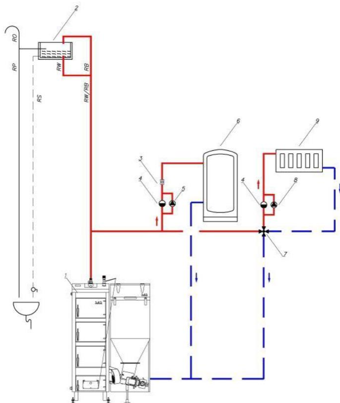
Abb. 5. Beispielschema der Schutzvorrichtungen für Wasserheizgeräte nach PN-91/B-02413 in einem offenen System
