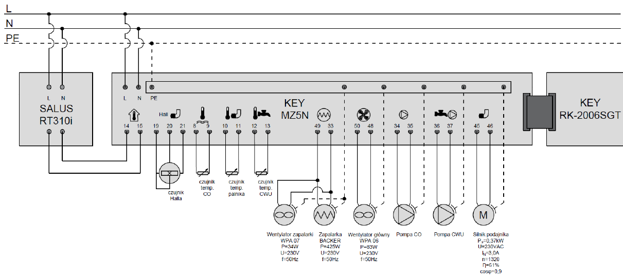
Abb. 8. Elektrischer Schaltplan des Kessels ECO QUENTIN 40 kW.
