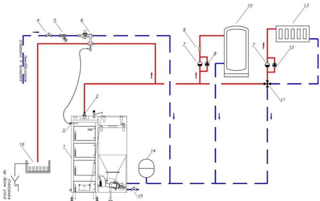
Abb. 6. Beispielschema der Schutzvorrichtungen für Wasserheizgeräte gemäß PN-EN 12828: 2013-05E in einem geschlossenen System.
