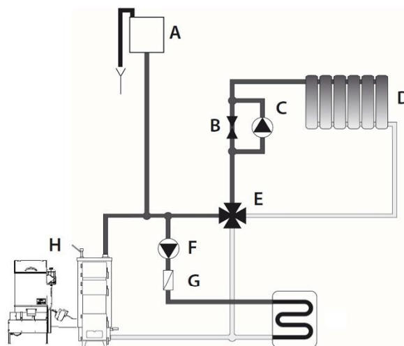
Abb. 2. Lage und Anschlussweise des Kessels in der Zentralheizungsinstallation des Hauses
