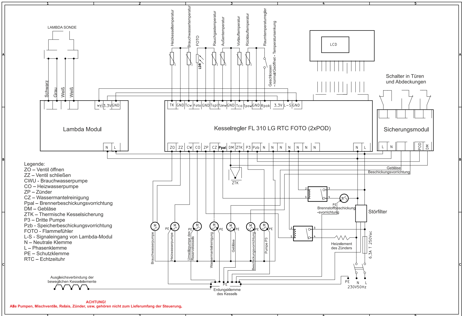
Zeichnung 10.1 Elektrisches Anschlussschema des Heizkessels
