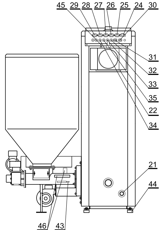
Zeichnung 7.1 Grundlegende Bauelemente des Heizkessels SD DUO / SD DUO BIO
