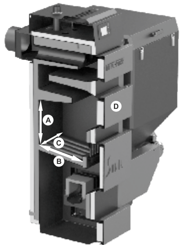
Zeichnung 7.3.2 Abmessungen der Nebenbrennkammer und der Einfüllöffnung des Heizkessels SD DUO BIO
