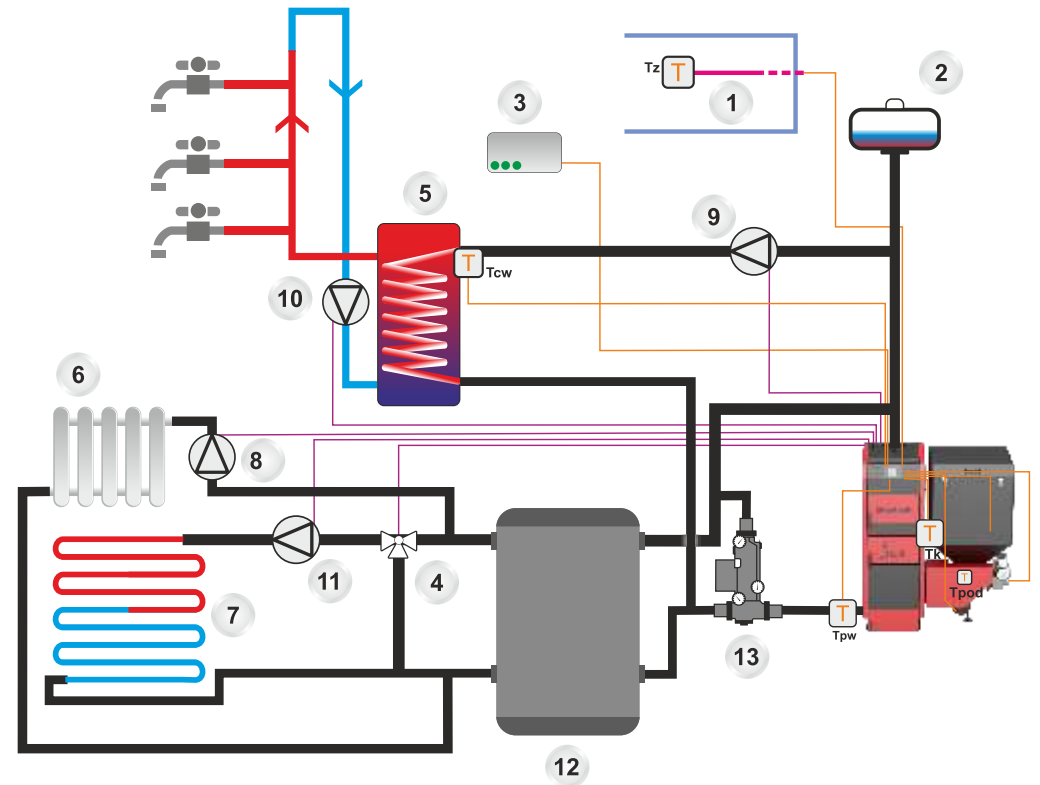
Zeichnung 8.2.4 Anschluss des Heizkessels an die Heizungsinstallation mit Laddomat und Pufferspeicher
