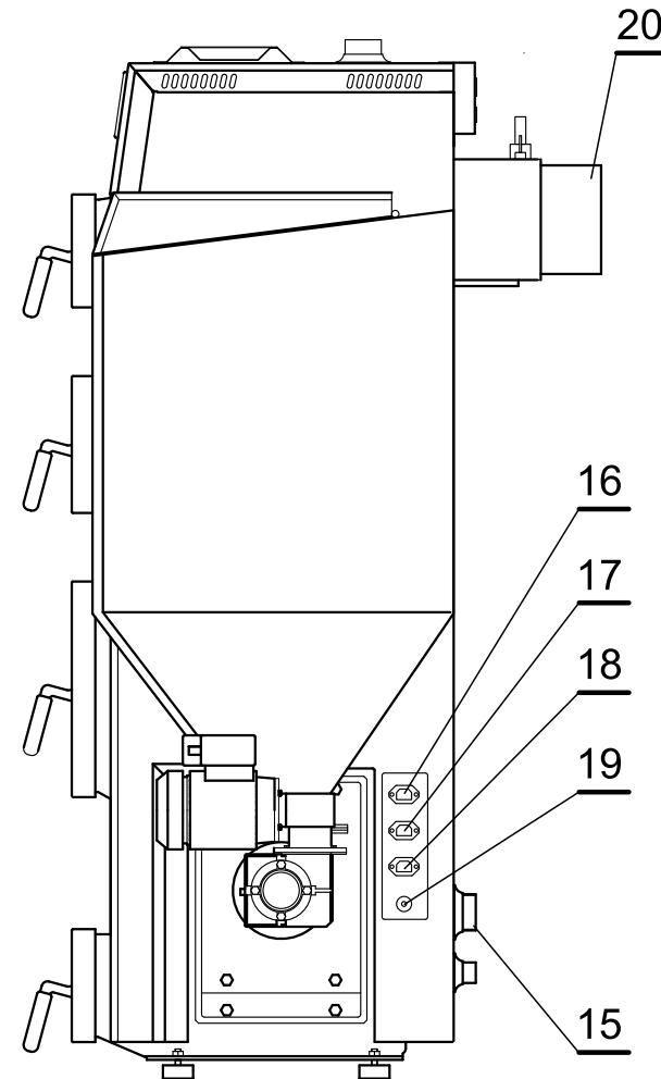
Zeichnung 7.1 Grundlegende Bauelemente des Heizkessels SD DUO / SD DUO BIO
