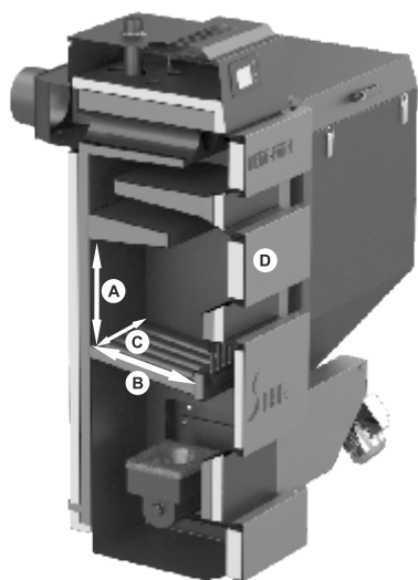
Zeichnung 7.2.2 Abmessungen der Nebenbrennkammer und der Einfüllöffnung des Heizkessels SD DUO
