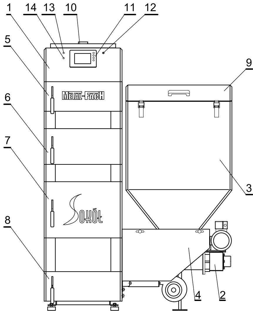
Zeichnung 7.1 Grundlegende Bauelemente des Heizkessels SD DUO / SD DUO BIO
