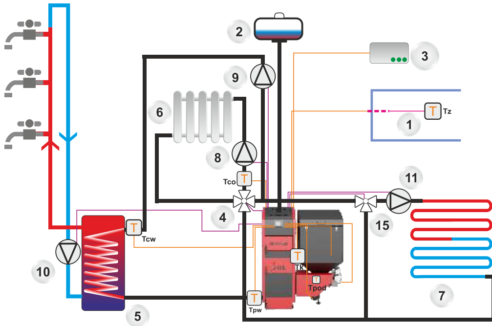
Zeichnung 8.2.3 Anschluss des Heizkessels an die Heizungsinstallation
