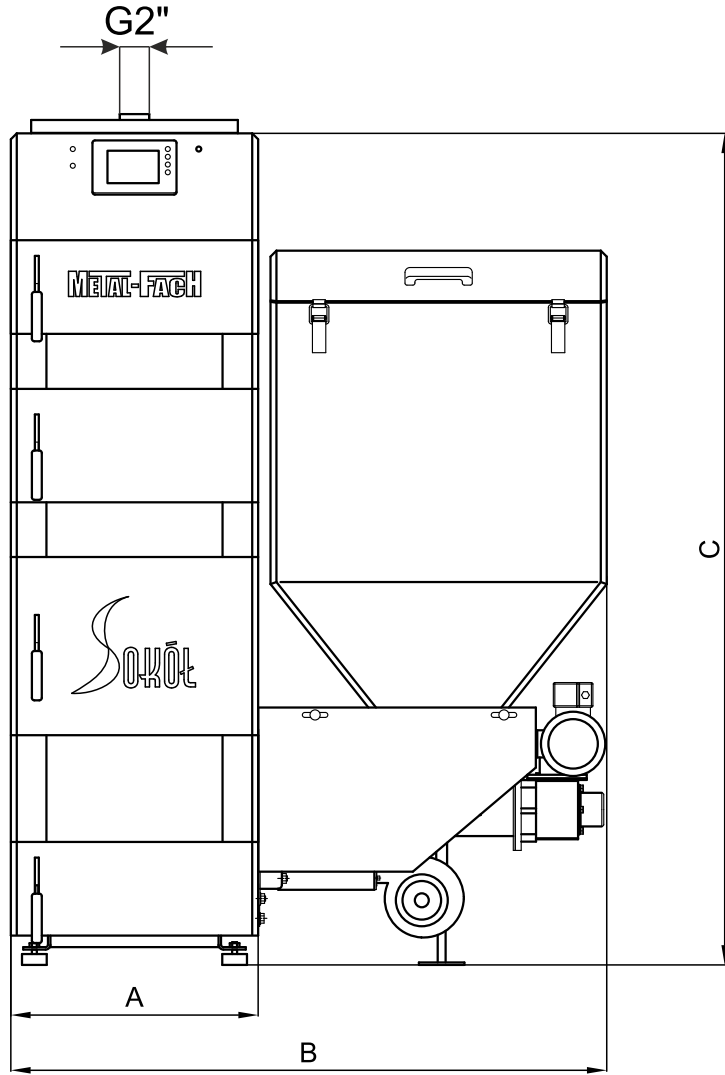
Zeichnung 7.3.1 Abmessungen des Heizkessels SD DUO BIO
