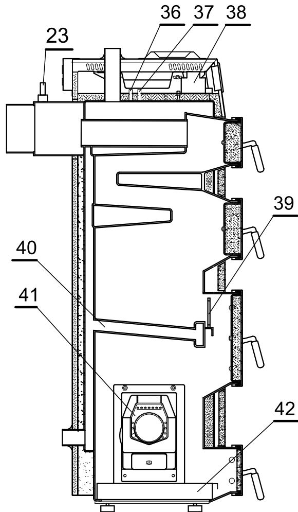
Zeichnung 7.1 Grundlegende Bauelemente des Heizkessels SD DUO / SD DUO BIO
