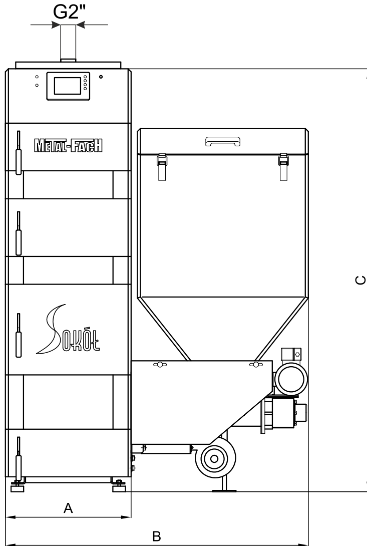
Zeichnung 7.2.1 Abmessungen des Heizkessels SD DUO
