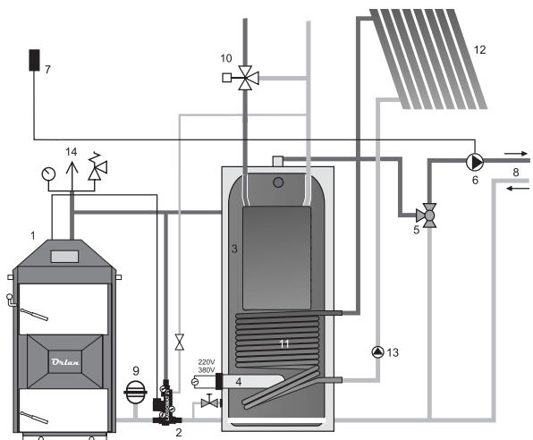
Bild 9. Das vorbildliche Schema des Anschlusses des Wärmespeichersystems mit einem von Speicher NADO mit eingebautem Gebrauchwassergefäß und mit Schlange und Sonnenkollektor.
