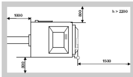
Bild 1. Aufstellung des Kessels Orlan.
