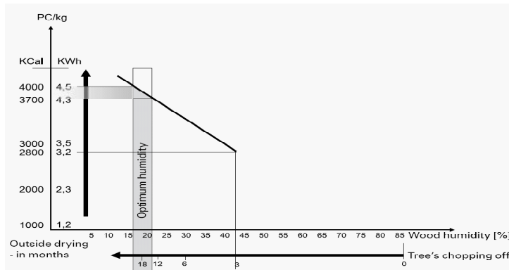
Bild 7. Holzfeuchtigkeit-Diagramm.
