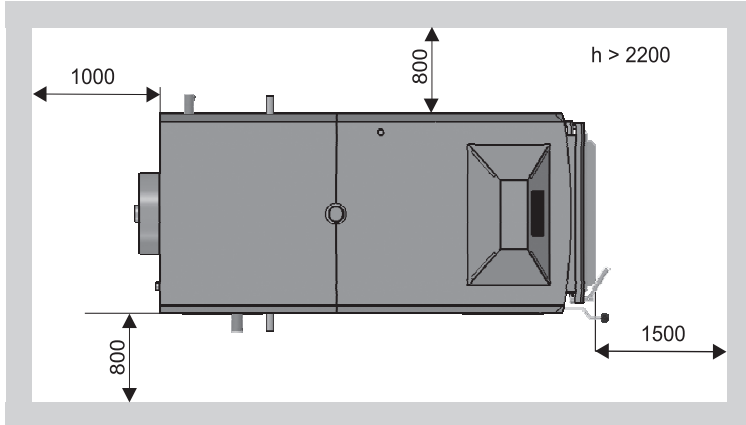
Abb.1 Aufstellung des ORLAN SUPER.
