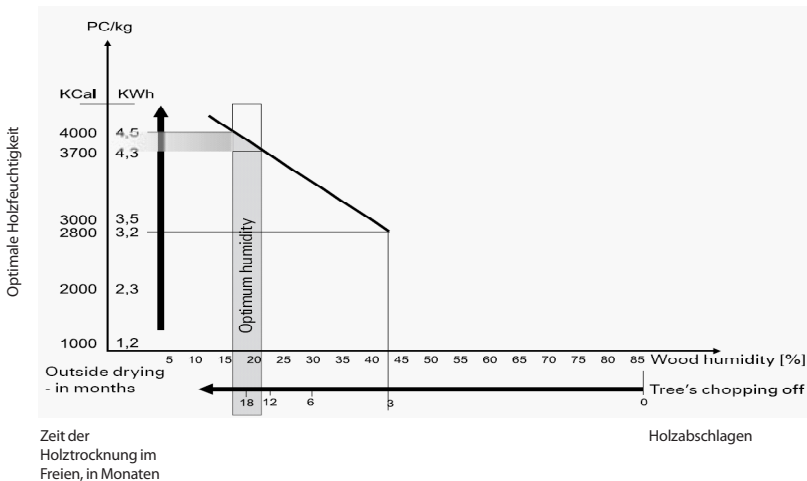
Abb.2 Diagramm zur Holzfeuchte
