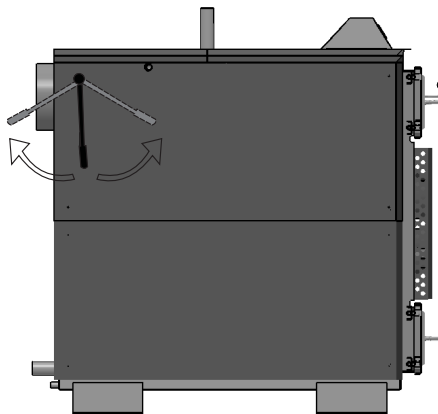
Abb. 4 Reinigung des Wärmetauschers mittels Hebel.
