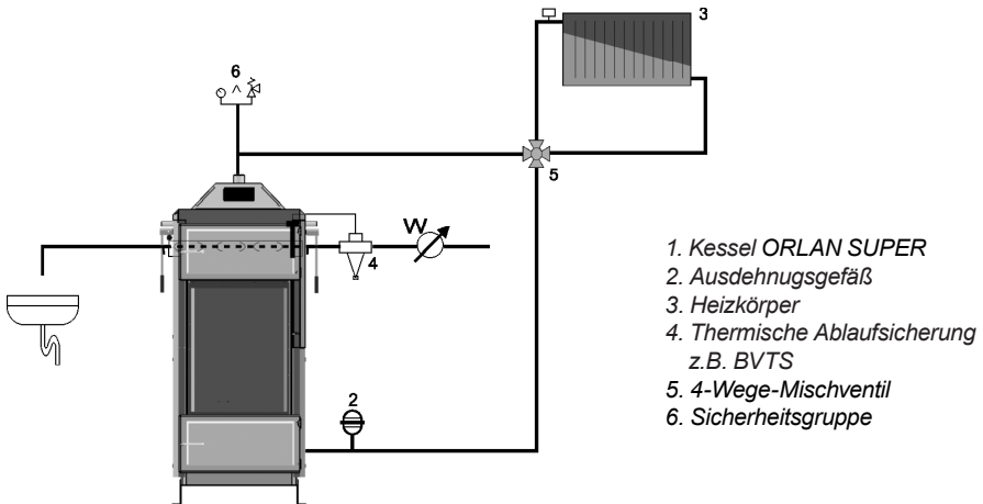
Abb.5 Anschluss der thermischen Ablaufsicherung (z.B. BVTS) des Kessels ORLAN SUPER.
