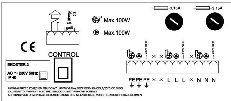
Abb.2 Blick von hinten auf die Regelung: Anschlussschema.
