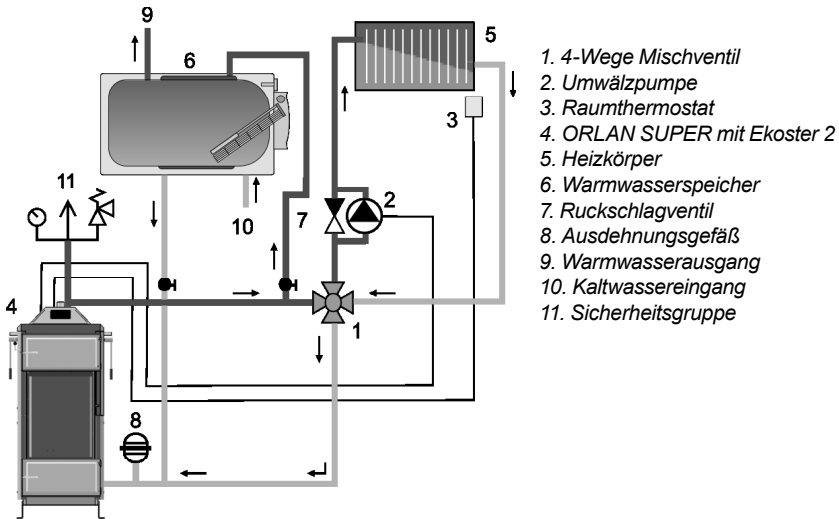
Abb.3 Anschluss-Schema mit dem Kessel ORLAN SUPER Und 4-Wege Mischventil
