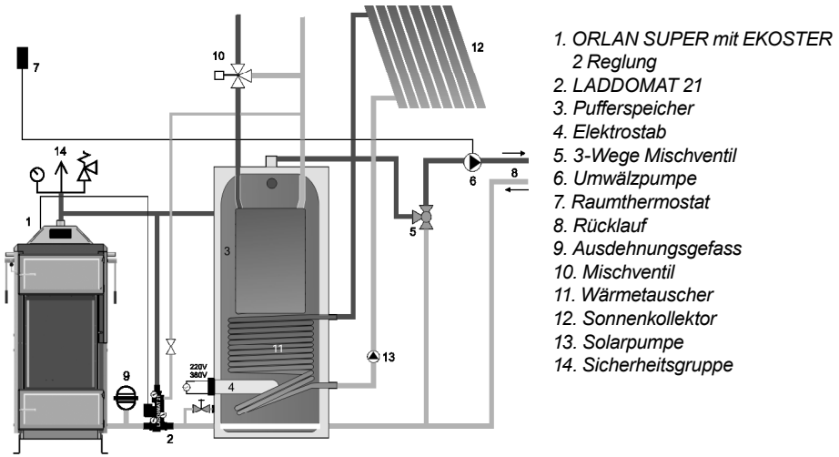
Abb4 Beispiel eines Anschluss-Schemas des Wärmetauschersystems mit einem Speicher mit eingebautem Brauchwassergefäß und Wärmetauscher Und Sonnenkollektor.
