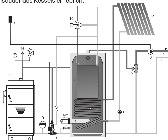
Bild 9. Anschlusschema des Wärmespeichersystems mit einem Kombispeicher (mit eingebautem Warmwasserbehälter und Wärmetauscher) und Sonnenkollektoren
