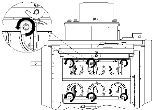
KROK 5. Poluzować śruby mocujące tuleje ramienia łącznika tak, aby możliwe było wysunięcie wałka z tulei mocujących ramiona łącznika.
