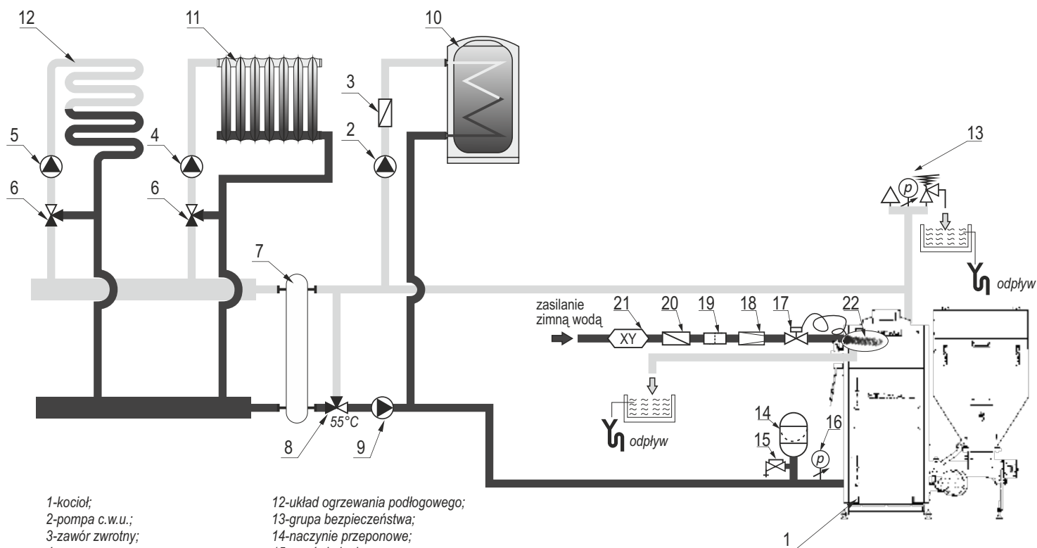
Rysunek 10. Przykładowy schemat instalacji grzewczej systemu otwartego.
