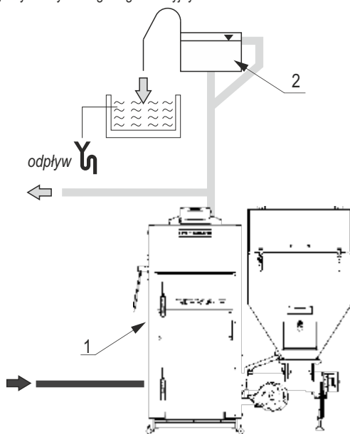
Rysunek 5. Przykładowy schemat zabezpieczeń kotła SIGMA E w układzie otwartym: 1-kocioł; 2-otwarte naczynie wzbiorcze.
