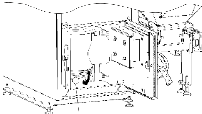
KROK 2. Wysunąć szufladę na popiół, oczyścić.
