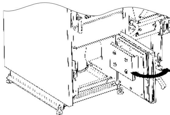
KROK 1. Otworzyć drzwi paleniskowo-popielnikowe.
