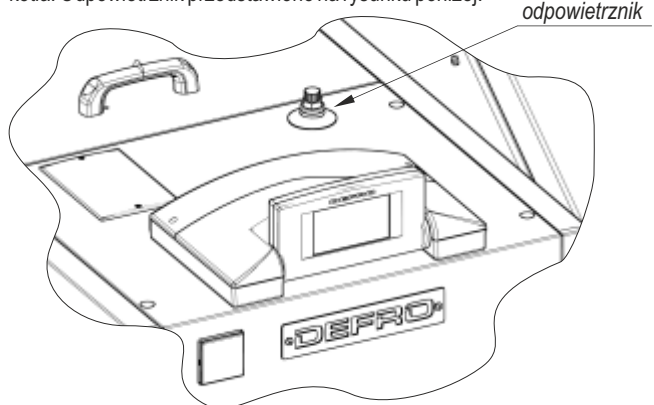
Rysunek 12. Odpowietrznik kotła.
