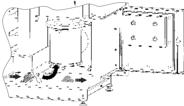
KROK 3. Za pomocą dostarczonych narzędzi odchylić klapę, przegarnąć popiół i usunąć przez drzwi paleniskowo-popielnikowe. Ponownie wsunąć szufladę i zamknąć drzwi
