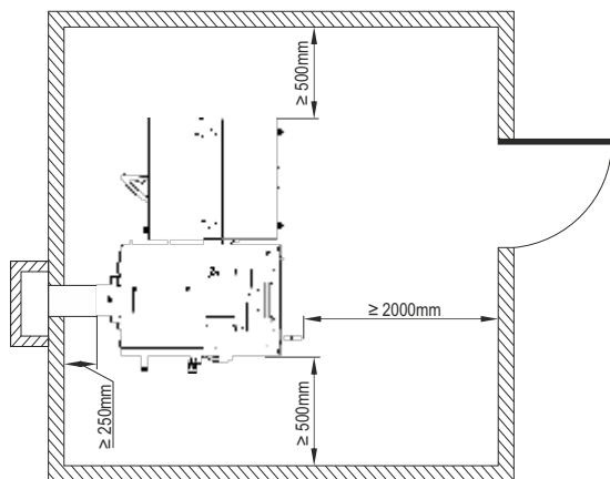
Rysunek 3. Ustawienie kotła w pomieszczeniu kotłowni.
