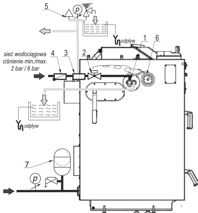
Rysunek 7. Przykładowy schemat zabezpieczeń kotła SIGMA NZ w układzie zamkniętym: 1-wężownica; 2-zawór BVTs wkręcony w wężownicę; 3-filtr wody użytkowej; 4-zawór zwrotny; 5-armatura bezpieczeństwa; 6-czujnik zaworu BVTs; 7-naczynie wzbiorcze przeponowe.
