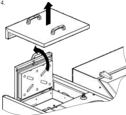
KROK 1. Podnieść osłonę maskującą i otworzyć drzwi wyczystne górne
