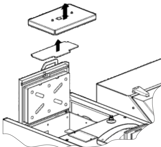
KROK 2. Wyciągnąć z kotła odbojnice spalin
