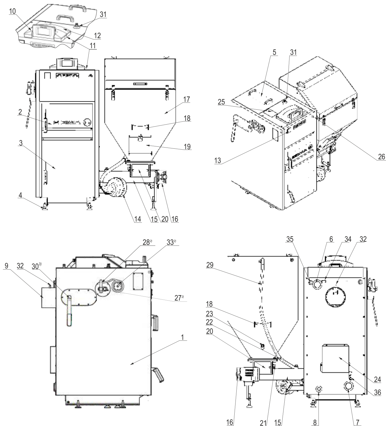
Rysunek 2. Podstawowe elementy kotłów.
