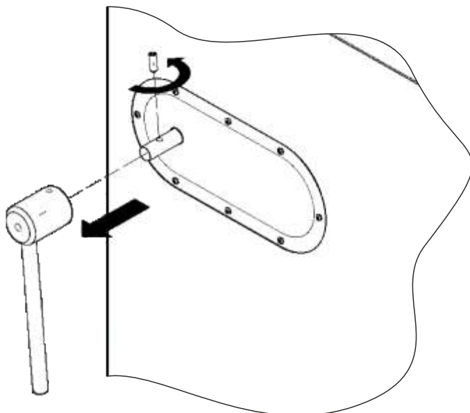
KROK 3. Odkręcić wkręt dociskowy imbus M8x25 mocujący rączkę mechanizmu czyszczącego i zdjąć ją z wałka mechanizmu.
