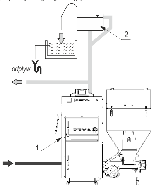
Rysunek 5. Przykładowy schemat zabezpieczeń kotła SIGMA w układzie otwartym: 1-kocioł; 2-otwarte naczynie wzbiorcze.
