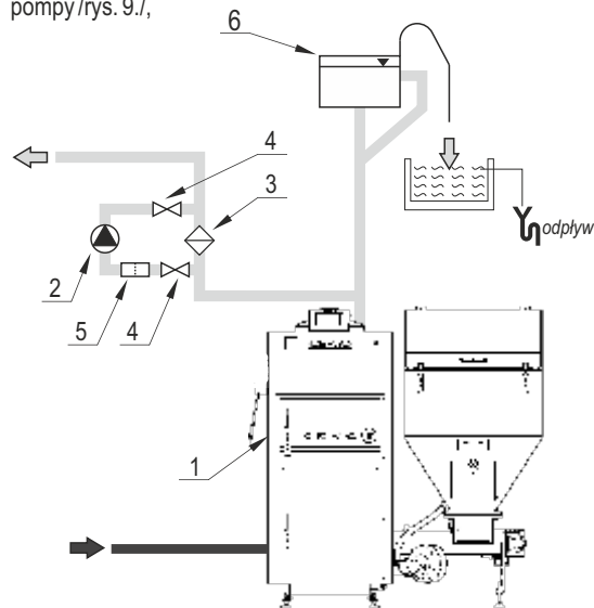
Rysunek 9. Wykonanie obejścia grawitacyjnego: 1-kocioł; 2-pompa obiegowa; 3-zawór różnicowy; 4-zawory odcinające; 5-filtr; 6-otwarte naczynie wzbiorcze.
