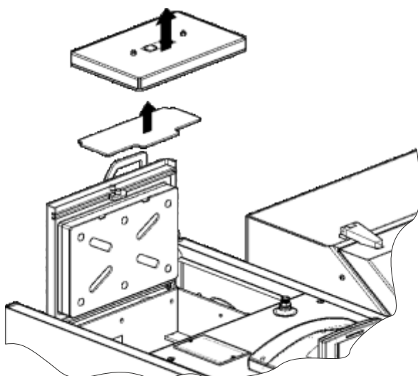
KROK 2. Wyciągnąć z kotła odbojnice spalin
