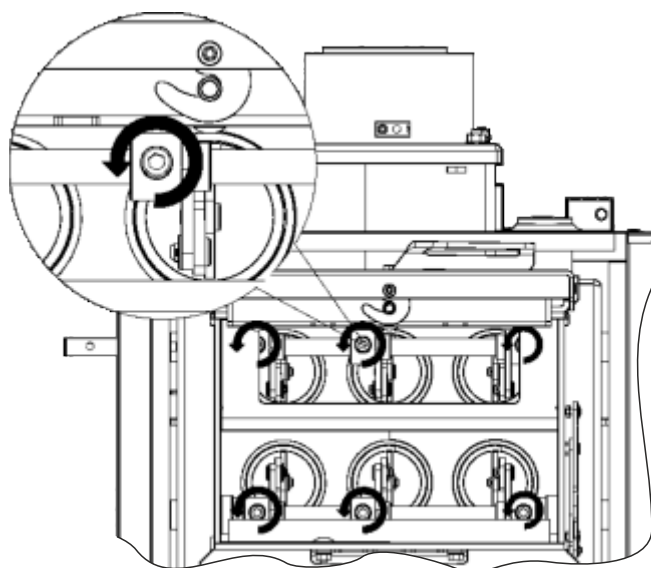
KROK 5. Poluzować śruby mocujące tuleje ramienia łącznika tak, aby możliwe było wysunięcie wałka z tulei mocujących ramiona łącznika.
