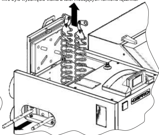
KROK 5. Stopniowo wysuwać wałek mechanizmu czyszczącego oraz pojedynczo wyciągać zawirowywacze. Czynność należy wykonywać ostrożnie w celu uniknięcia „opadnięcia” zawirowywaczy w głąb rurowych ciągów spalinowych. Zdemontowane zawirowywacze, skontrolować i przeczyścić za pomocą twardej szczotki dostarczonej wraz z kotłem. Ponowne zmontować mechanizm czyszczący w odwrotnej kolejności. W kotłach o mocy 24-48 kW zasada demontażu zawirowywaczy jest analogiczna jak w opisanym przykładzie z tym, że zastosowano dwa wałki mechanizmu czyszczącego. Różnica polega na dodatkowym demontażu cięgna łączącego wałki.
