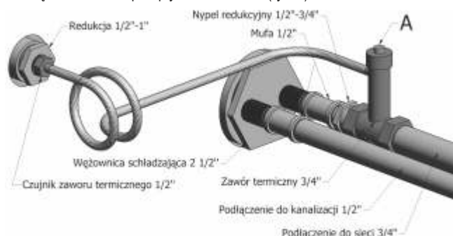
Rysunek 6. Sposób podłączenia termicznego zabezpieczenia odpływu.
