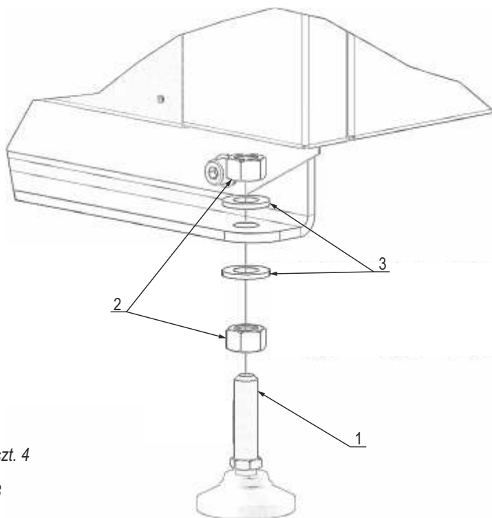
Rysunek 15. Sposób montażu stopek ustalających kocioł.
