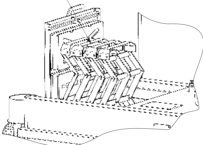
Rysunek 12. Zawirowywacze w kotle.
