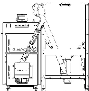
Rysunek 10. Prawidłowe ustawienie zasobnika paliwa względem kotła.
