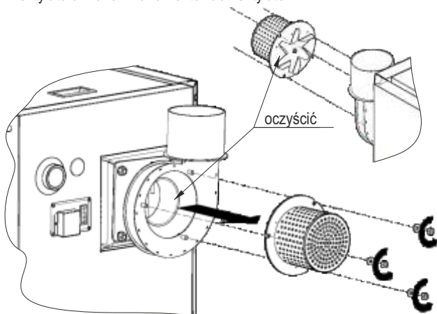
Rysunek 14. Sposób oczyszczania wentylatora wyciągowego.
