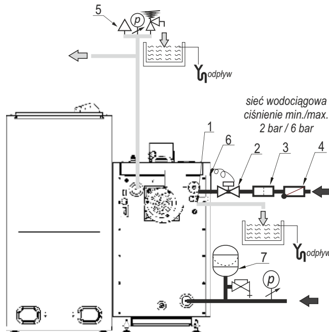
Rysunek 5. Przykładowy schemat zabezpieczeń kotła SMART EKOPELL w układzie zamkniętym: 1-wężownica; 2-zawór BVTS wkręcony w wężownicę; 3-filtr wody użytkowej; 4-zawór zwrotny; 5-armatura bezpieczeństwa; 6-czujnik zaworu BVTS; 7-naczynie wzbiorcze przeponowe.
